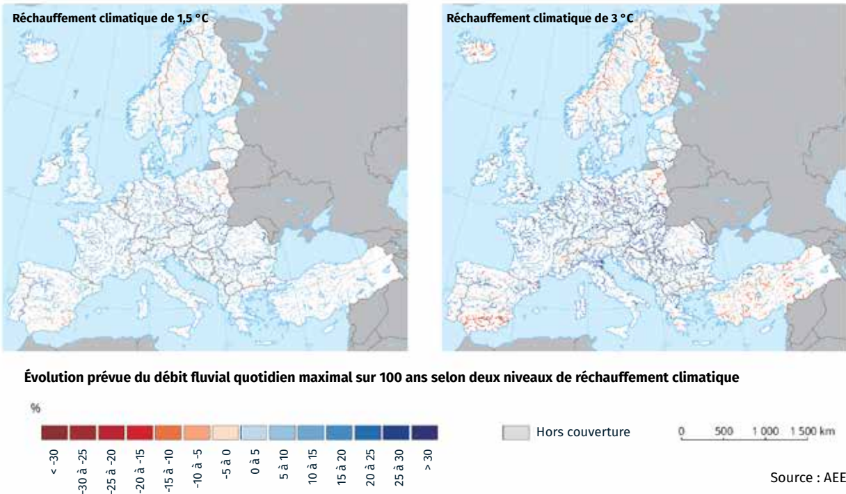
Fig. 14 - Évolution prévue du débit fluvial quotidien maximal sur 100 ans selon deux niveaux de réchauffement climatique (1,5 °C et 3 °C) 49
