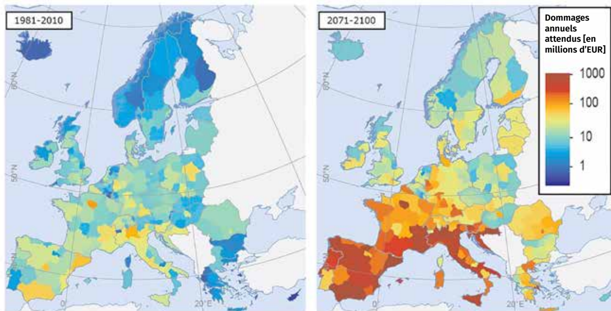
Fig. 5 - Dommages annuels attendus subis par les infrastructures critiques européennes en raison des aléas naturels globaux liés au changement climatique 14
