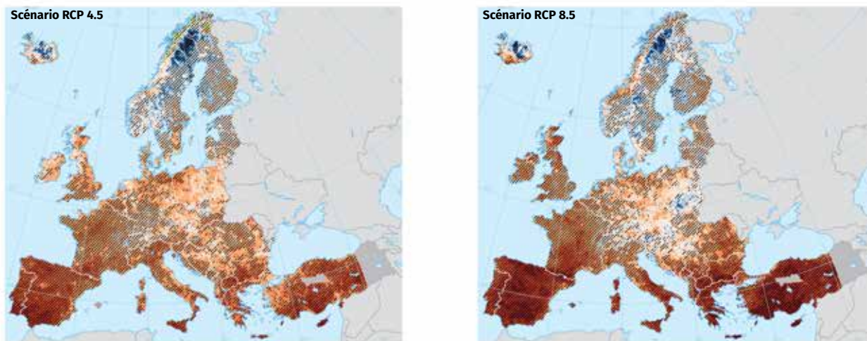
Évolution prévue de la fréquence des sécheresses météorologiques entre 1981 - 2010 et 2041 - 2070 selon deux scénarios climatiques
